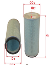
A-5417 ES-11056
